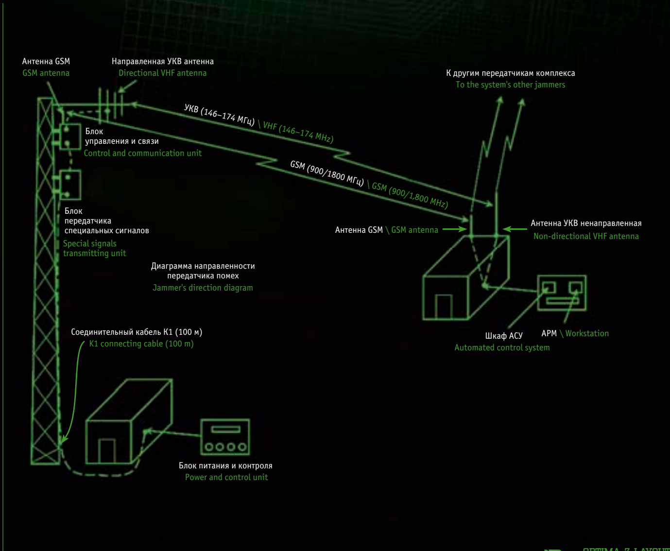
OPTIMA-3 LAYOUT
